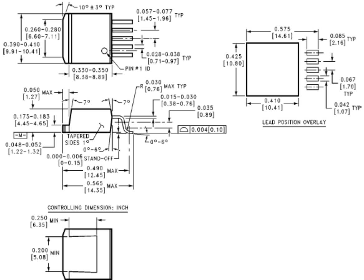
TO-263 封装 (S) 尺寸图 单位：英寸/毫米
