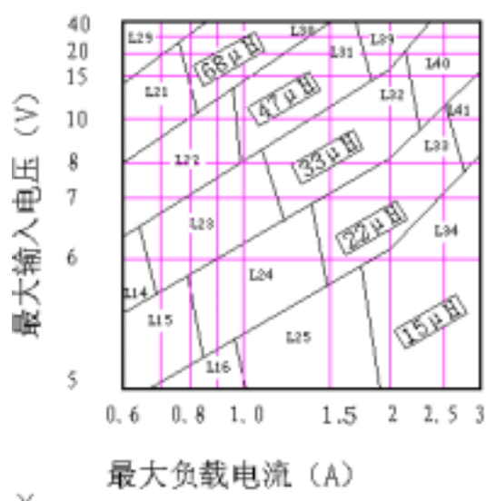
图 4 LM2596 —3.3
